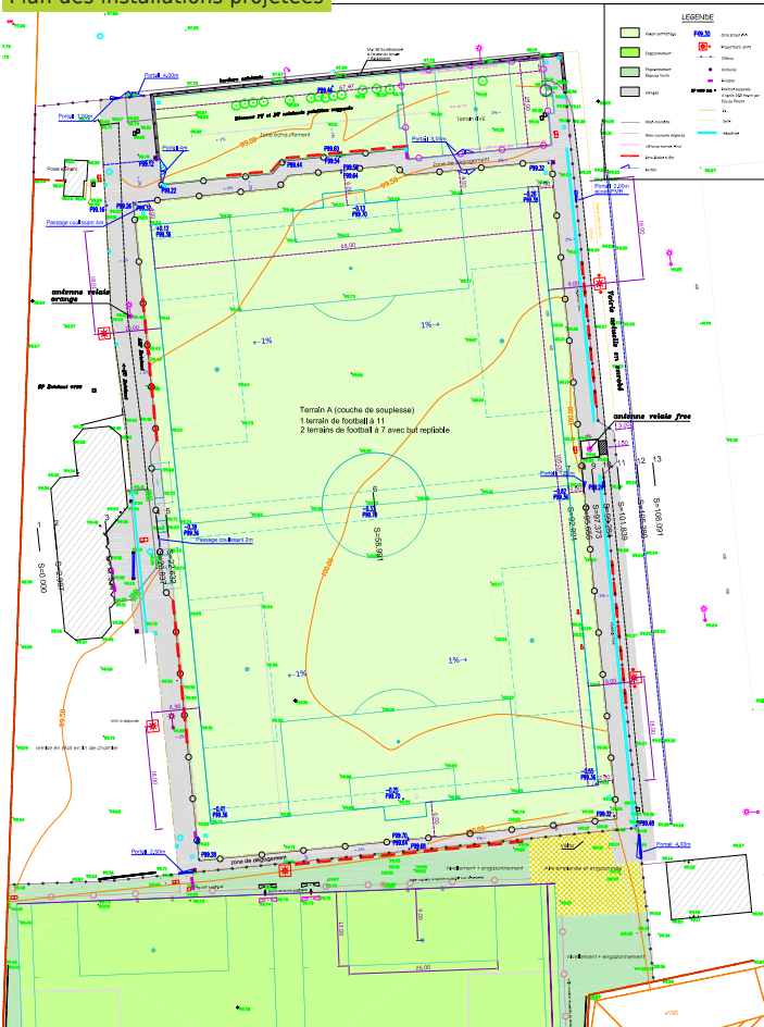
Plan des installations projetées
