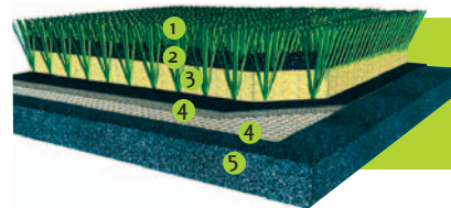
Schéma de composition du gazon
